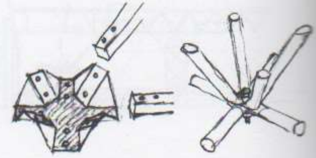
Unistrut. Lámina estampada forma nudo
