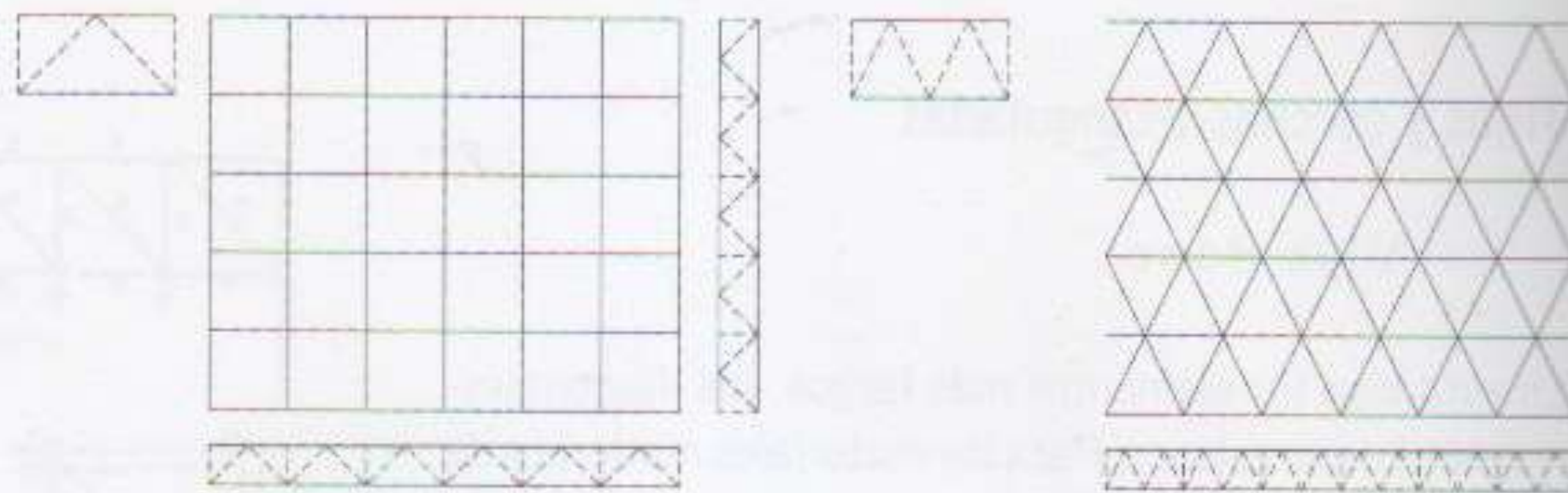
Fig 60a Tipos de tramas estereométricas
