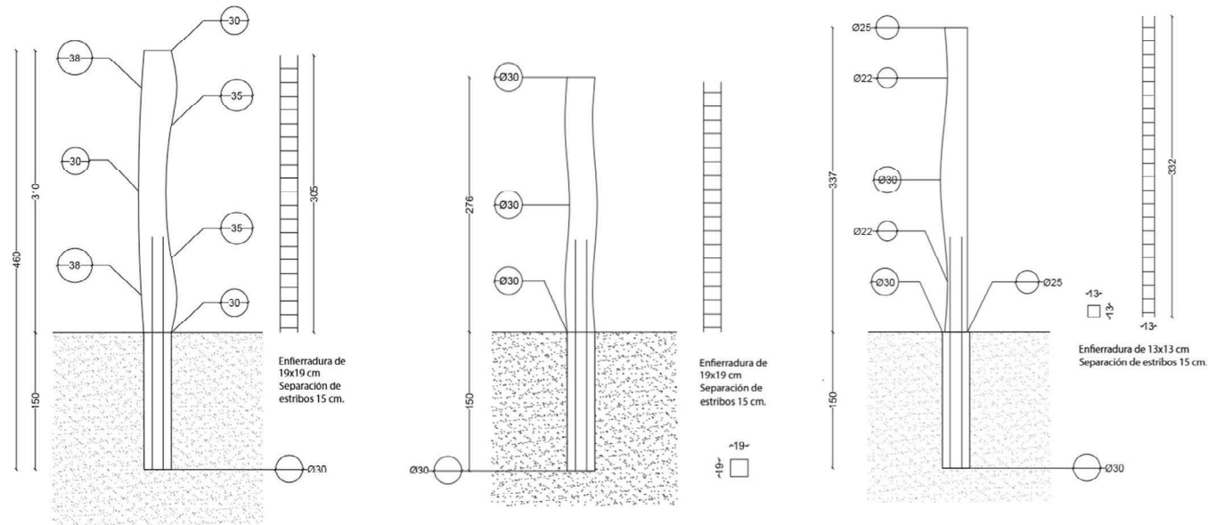
Figura 9. Análisis estructural de los modelos (arriba), generación de trazados de ejecución y estructura (abajo). Fuente: Elaboración propia.
