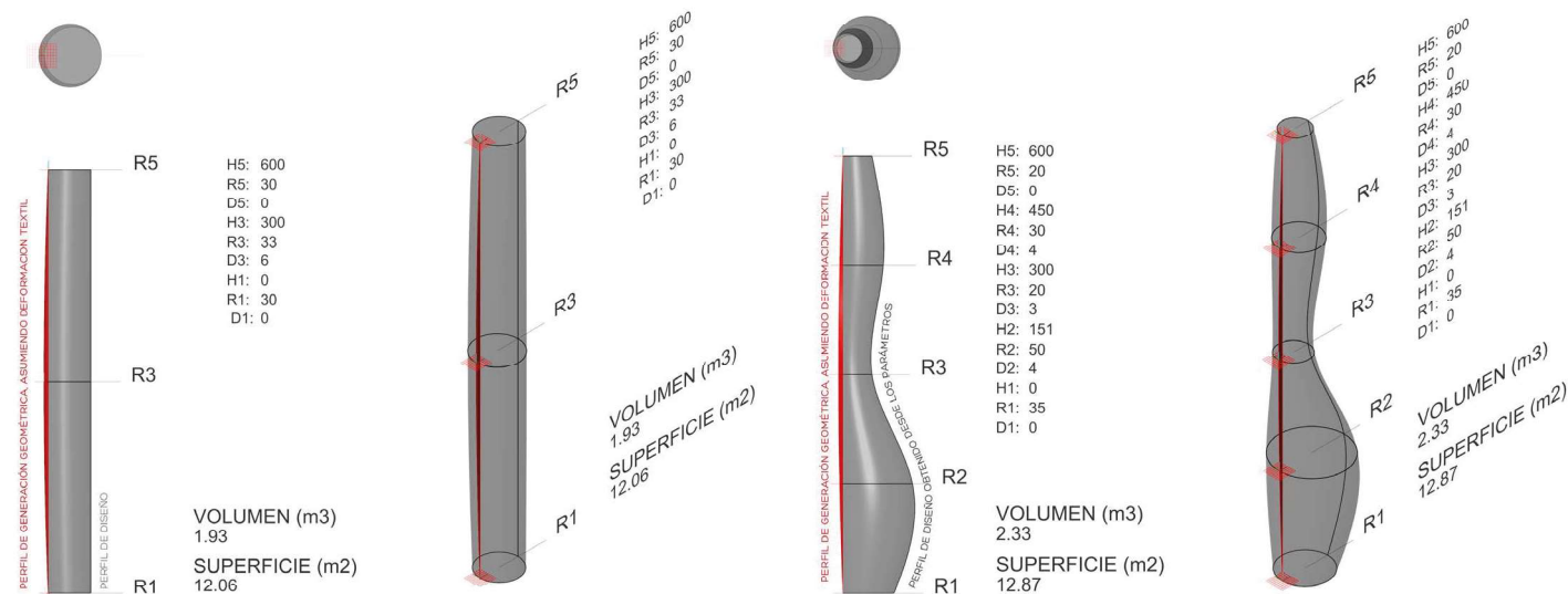
Figura 3. Generación de columnas según diferentes valores paramétricos. Fuente: Elaboración propia.
