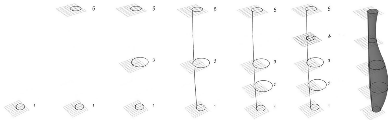
Figura 2. Programación paramétrica en Grasshopper (arriba) y estrategia de definición geométrica por circunferencias en un eje vertical (abajo). Fuente: Elaboración propia.
