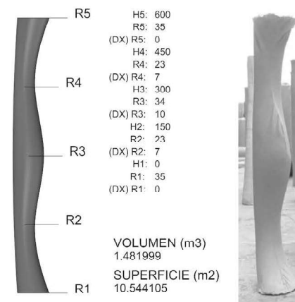
Figura 5. Comparación de modelos generados con la programación y columnas ejecutadas. Fuente: Elaboración propia.
